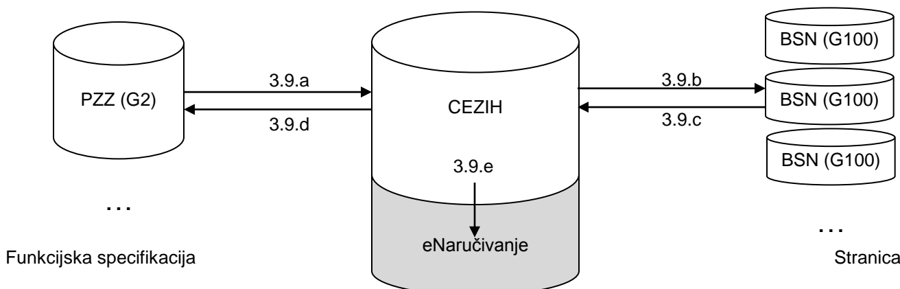
Slika 3.9: Tokovi informacija za rezervaciju termina
