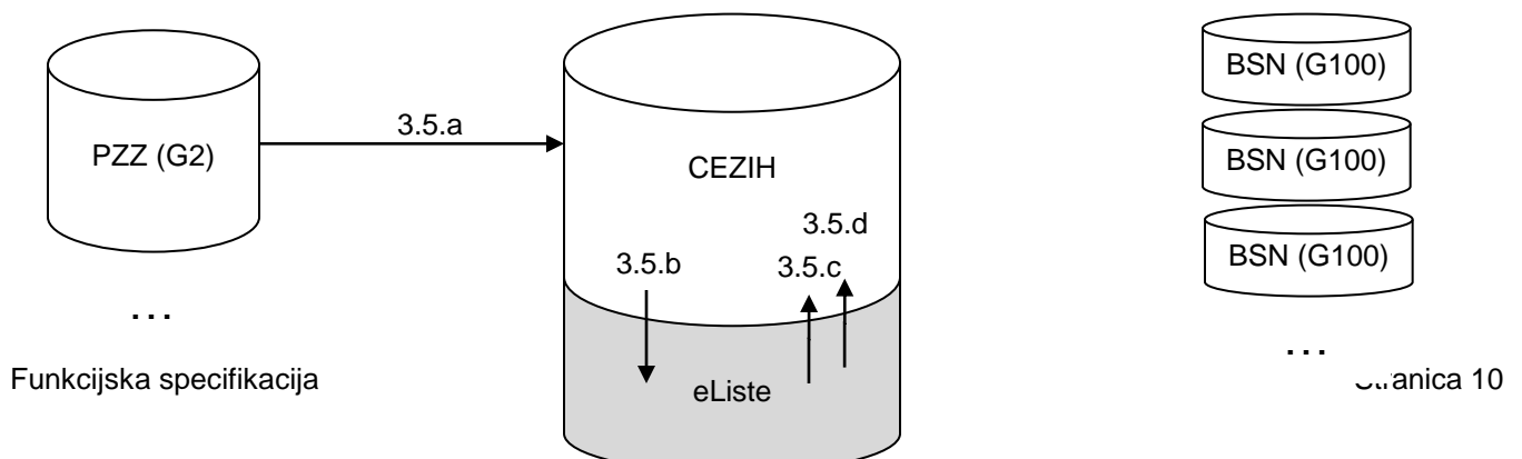
Slika 3.1: Tokovi informacija za dohvat prvog slobodnog blok termina kroz PZZ aplikaciju
